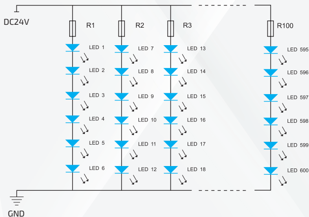
SCHAKELSCHEMA
