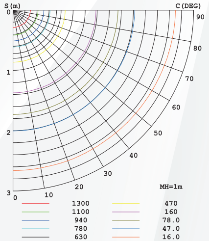
VLAKKE ISOLUX-DIAGRAM (EENHEID: 1X)
