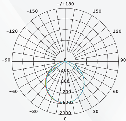
LICHTSTERKTEVERDELING DIAGRAM
